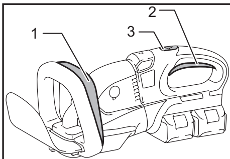
► 1. Gatillo interruptor B 2. Gatillo interruptor A 3. Botón lock-off (bloqueo desactivado)
