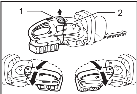
► 1. Knob 2. Housing
