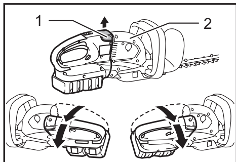
► 1. Perilla 2. Carcasa
