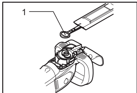
► 1. Orificio ovalado de las cuchillas de cizalla
