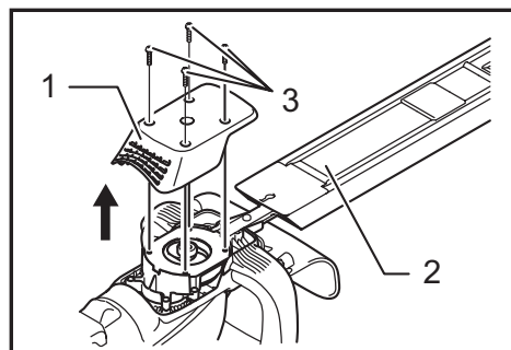
► 1. Sous-couvercle 2. Couvercle de lame 3. Vis
